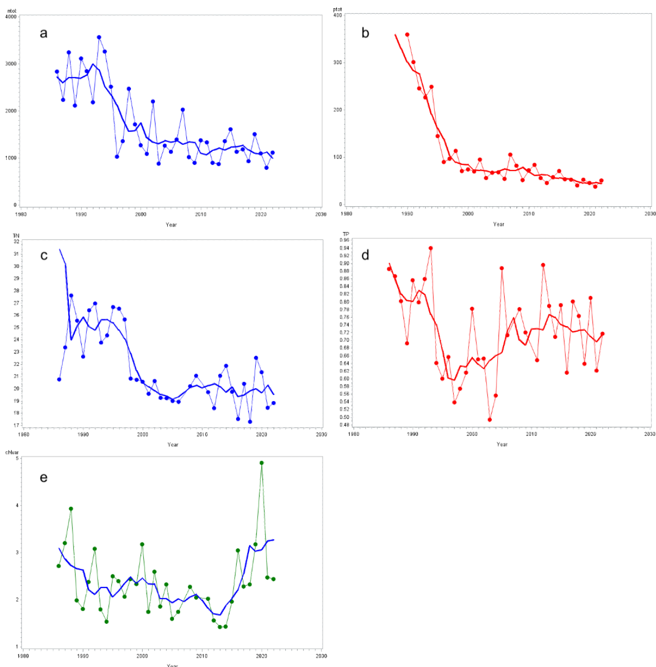
Figur 1.1. Tidslig udvikling i tilførsler af kvælstof i tons/år (a), fosfor tons/år (b) og koncentrationer af total kvælstof i µmol/l (c), total fosfor µmol/l (d) og klorofyl µg/l (e) for NOVANA station 1722 i Køge Bugt. Den markerede linje repræsenterer et 5 års glidende gennemsnit.
